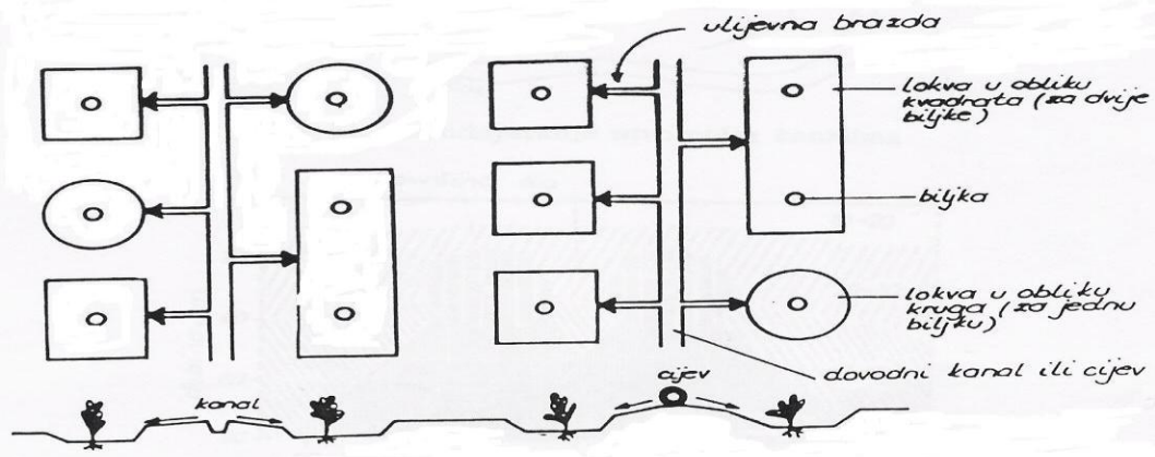
Prelievanje ili potapanje lokvama (tlocrt)
