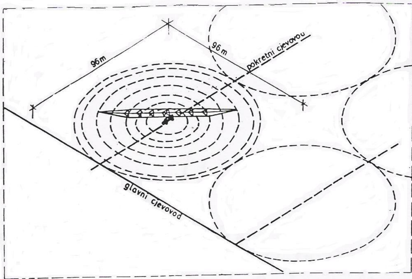
Skica navodnjavanja pomoću kružne prskalice («Bum sistem»)
