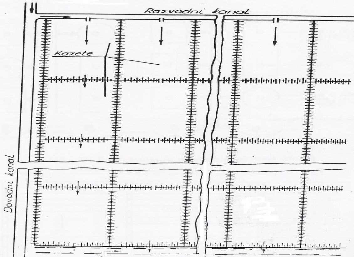
Preljevanje poprijeko na dužu stranicu parcelice (dvosmjerno prelijevanje)
