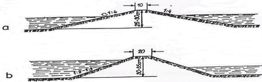
Presjek poprečnog (a) i uzdužnog (b) nasipa
