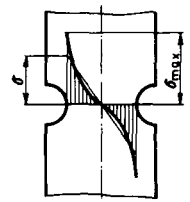
Razdioba naprezanja pri savijanju
