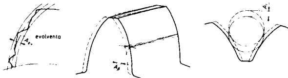
Tolerancije kružnog toka T_T
