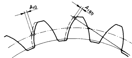
Granična odstupanja pri osnovnom koraku bokova zubača
