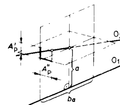
a – razmak osi b_a – aktivna širina zupčanika O_1, O_2 – osi
